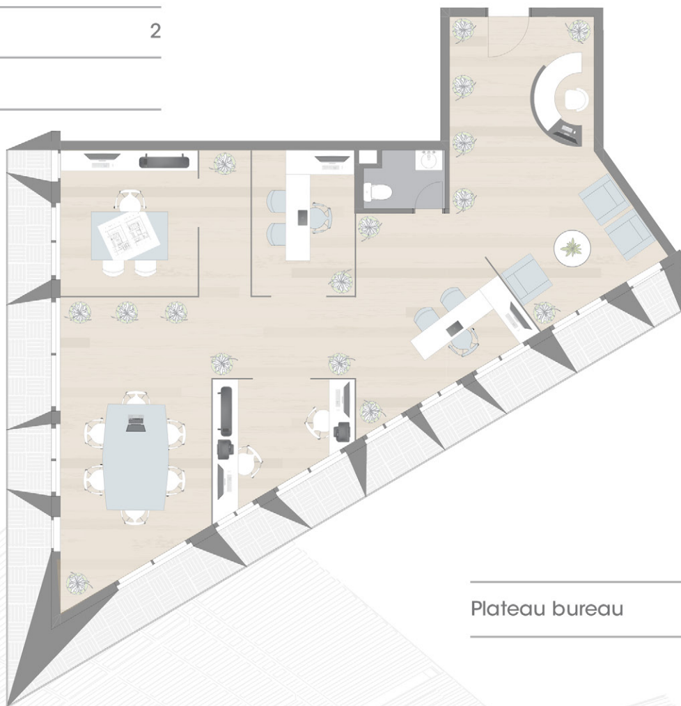
PLAN ETAGE 2
